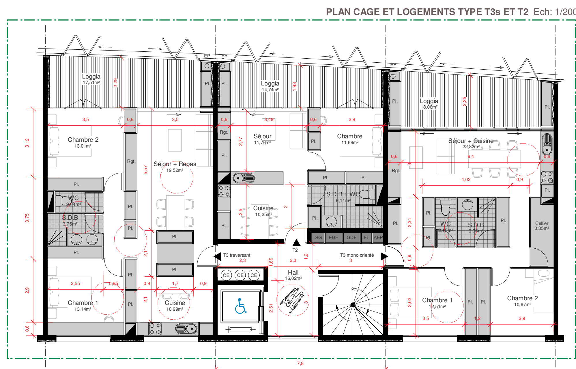
PLAN CAGE ET LOGEMENTS TYPE T3s ET T2 Ech: 1/200
