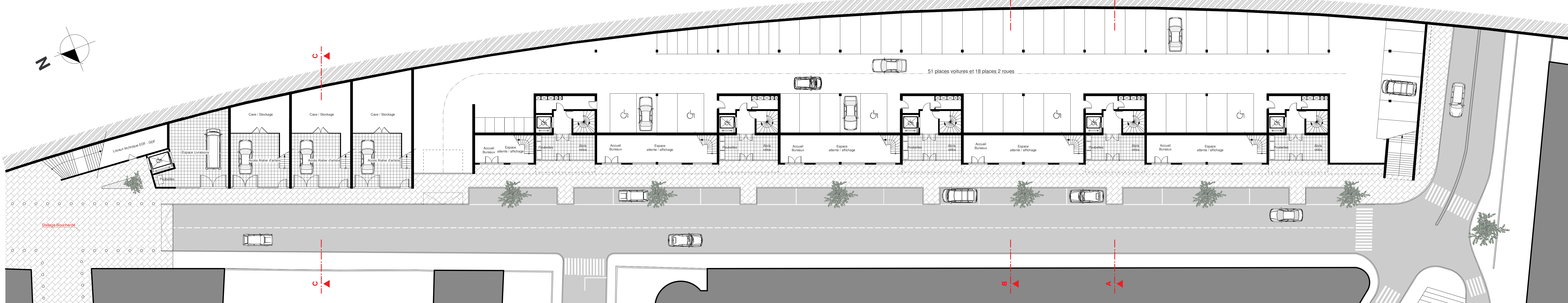
PLAN RDC (rue du Guesclin) Ech: 1/200
